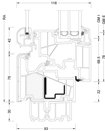
Senkrecht / Vertical
