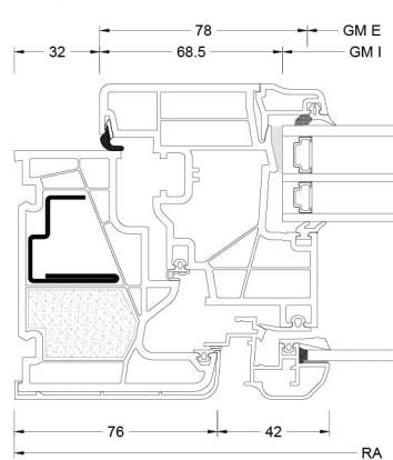
Waagrecht / Horizontal
